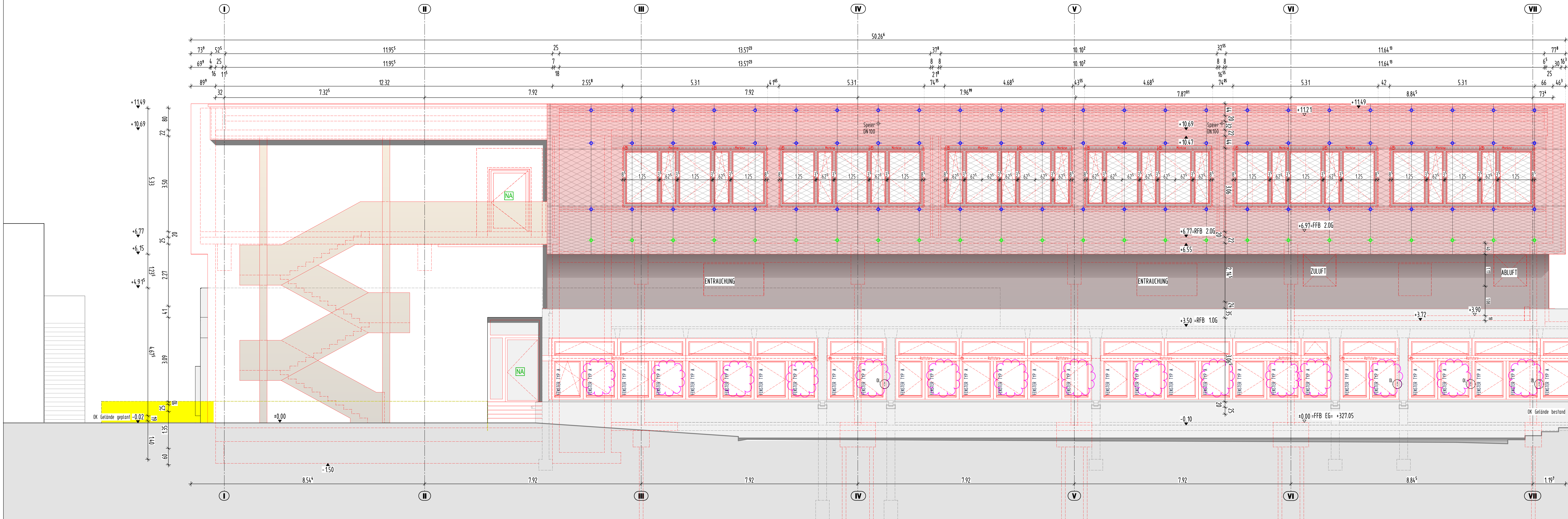
ANSICHT WEST BA1 M 1:50
