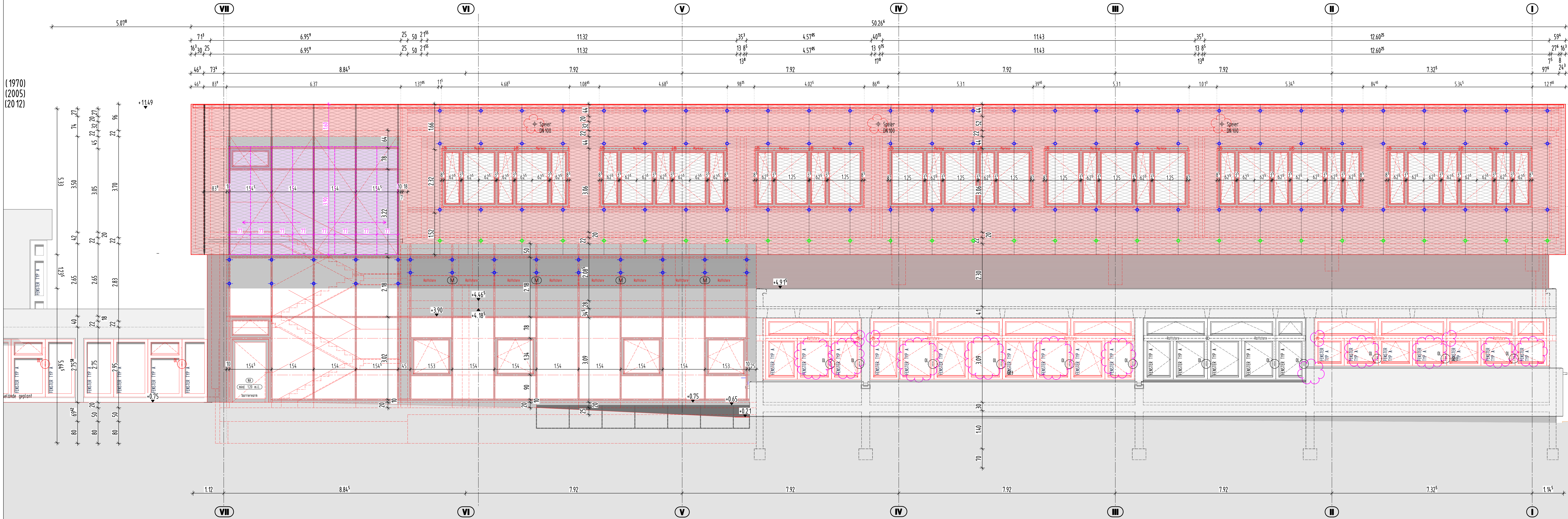
ANSICHT OST BA1 M 1:50
